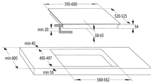
VDIT 661 C
