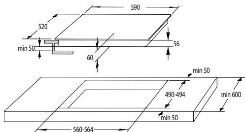
VDIT 630 C
