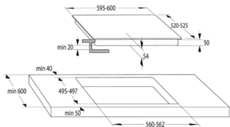
VDIT 652, 654, 657, 658, VDIS 658
